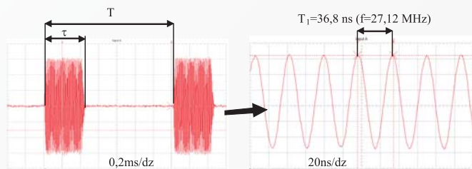
Rys. Z2. Przykładowa rejestracja oscyloskopowa modulowanego impulsowo pola elektromagnetycznego (MI) wytwarzanego przez diatermie fizykoterapeutyczną krótkofalową z głowicą zabiegową indukcyjną (współczynnik wypełnienia sygnału D = t/T=0,32 )
