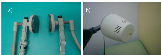
Rys. Z1. Przykłady aplikatorów zabiegowych stosowanych w diatermiach fizykoterapeutycznych krótkofalowych: a) pojemnościowy z okładkami sztywnymi okrągłymi; b) indukcyjny (fot. autorzy)
