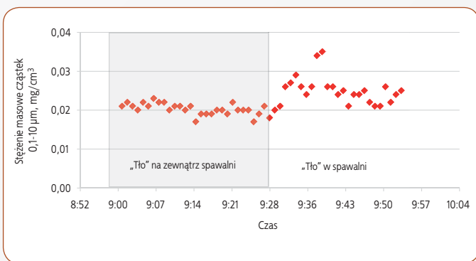
Rys. 5. Stężenie masowe cząstek z zakresu 0,1-10 µm w powietrzu atmosferycznym („tło” na zewnątrz spawalni) oraz w powietrzu w spawalni („tło” w spawalni) przed rozpoczęciem spawania (pomiar DUST-TRAK)
