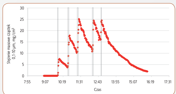
Rys. 6. Stężenie masowe cząstek z zakresu 0,1-10 µm w powietrzu na zewnątrz spawalni oraz w powietrzu w spawalni przed rozpoczęciem spawania, w trakcie spawania (tab. 1. – szare słupki wskazują czas 5 kolejnych operacji spawania) i po jego zakończeniu (pomiar DUST-TRAK)
