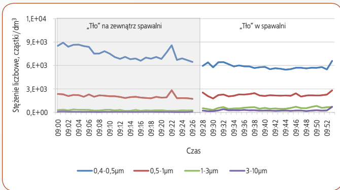
Rys. 3. Stężenie liczbowe cząstek z zakresu 0,4-0,5 µm, 0,5-1 µm, 1-3 µm i 3-10 µm w powietrzu atmosferycznym („tło” na zewnątrz spawalni) oraz w powietrzu w spawalni („tło” w spawalni) przed rozpoczęciem spawania (pomiar GRIMM)
