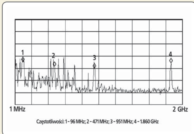
Rys. 1. Typowa charakterystyka widmowa pola elektrycznego z zakresu radiofalowego w pomieszczeniach biurowych na terenie Warszawy: 1 – pasmo UKF/FM, 2 – pasmo TV, 3 – pasmo GSM, 4 – pasmo DCS
