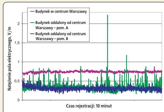
Rys. 2. Typowa charakterystyka zmienności pola elektrycznego z zakresu radiofalowego 100 kHz – 3 GHz, w 3 wybranych pomieszczeniach pracy biurowej na terenie Warszawy
